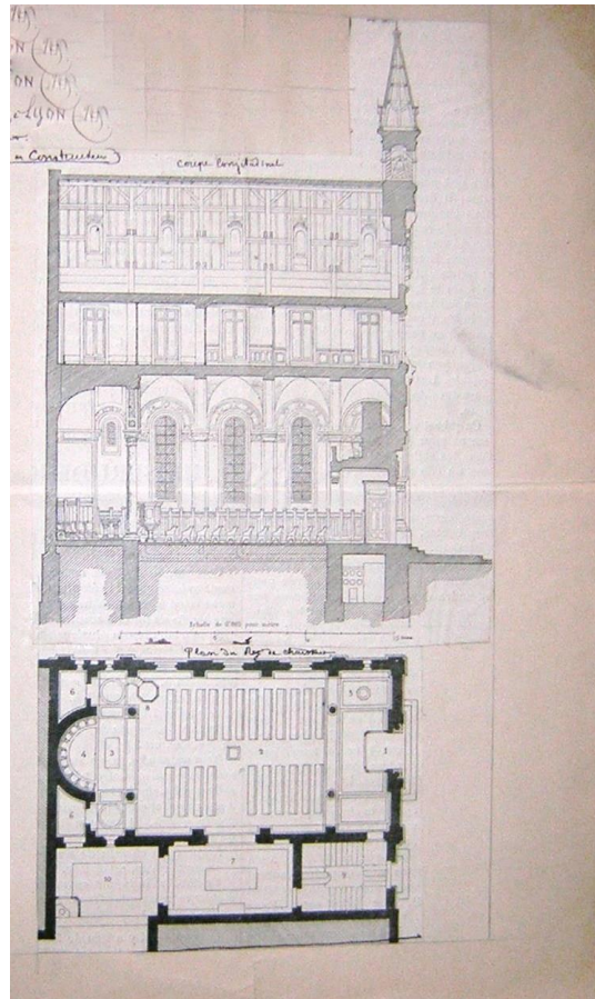
71-Coupe et plan de l'église
